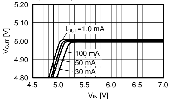
S-L2980A50 (Ta=25°C)
