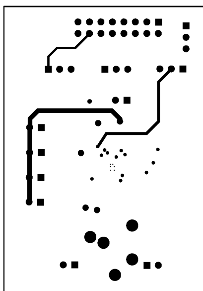
Figure 45. Bottom Layer
