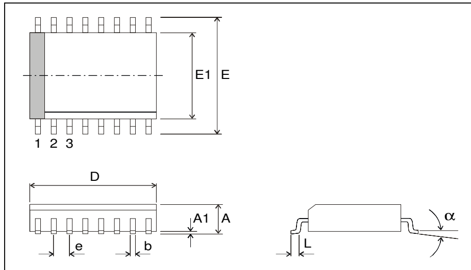
Fig. 2: QSOP16
