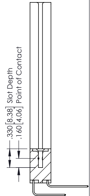
SECTION A-A
