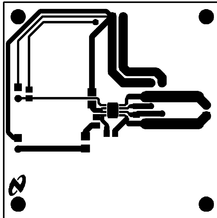
Figure 49. Top Layer
