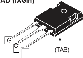
TO-268 (IXGT)
