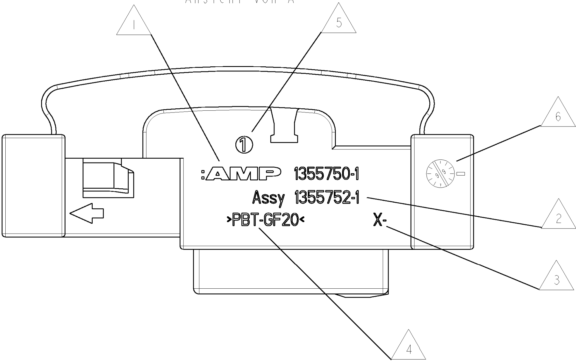
VIEW A Ansicht von A
