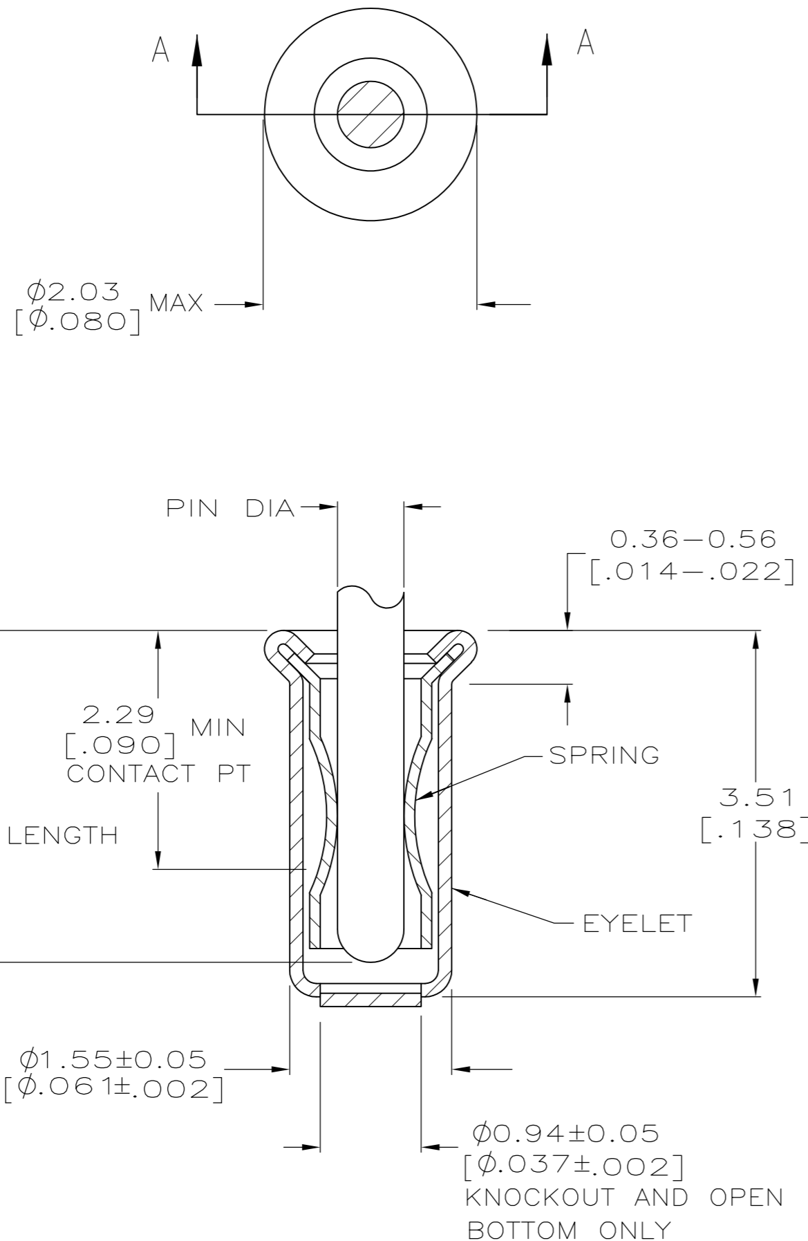
SECTION A-A
