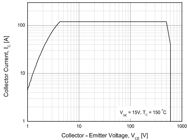
Fig. 15 RBSOA
