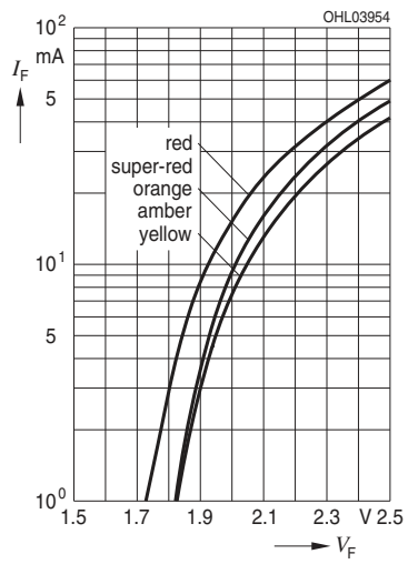
Forward Current 7) page 20 Durchlassstrom 7) Seite 20 I_F = f(V_F); T_A = 25\text{ °C}
