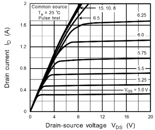
Fig. 8.2 I_D - V_{DS}
