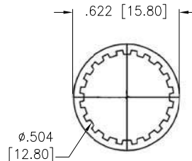
1/2-28UNEF-2B
