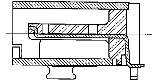
A-A (10:1) (CONTACT No. 1, 10)
