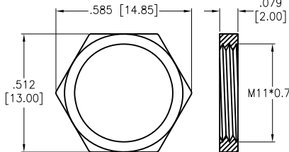
NUT
