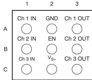
YHC PACKAGE WCSP 9-BALL (TOP VIEW)
