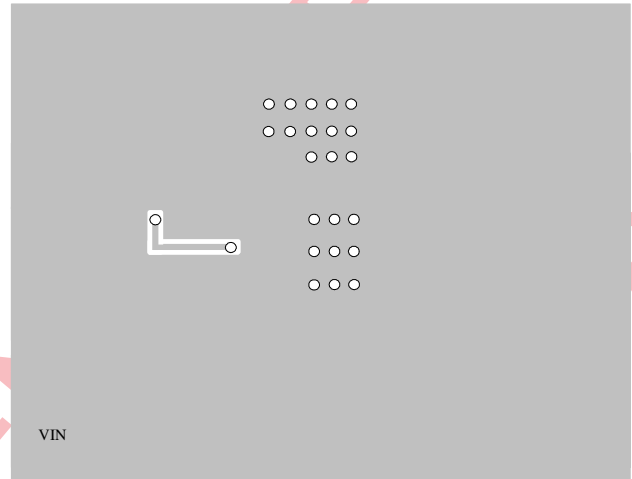
Bottom Layer
