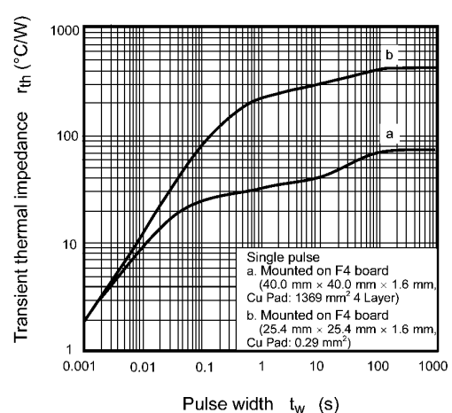
Fig. 7.12 r_{th} - t_w
