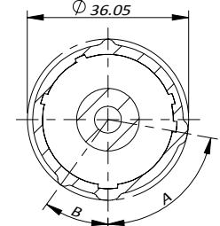
剖面 B-B 比例 1 : 1.5
