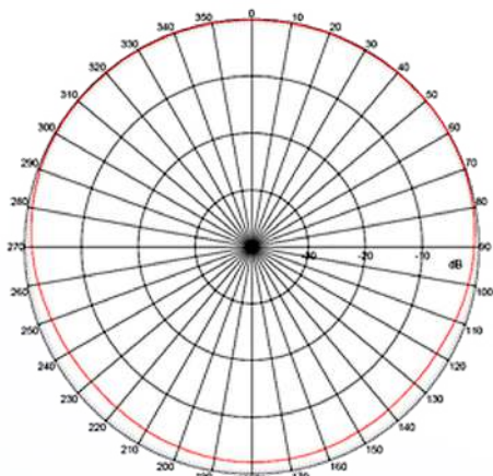
H-plane 5.5 GHz
