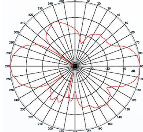
E-plane 5.5 GHz
