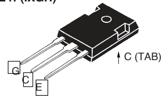
TO-268 (IXGT)
