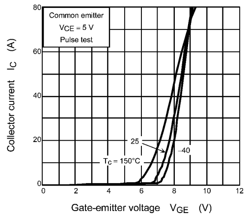
Fig. 8.6 I_C - V_{GE}
