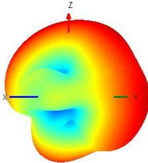
LTE 960MHZ
