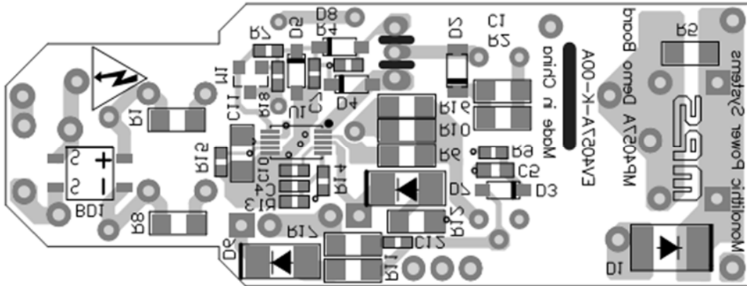
Bottom layer
