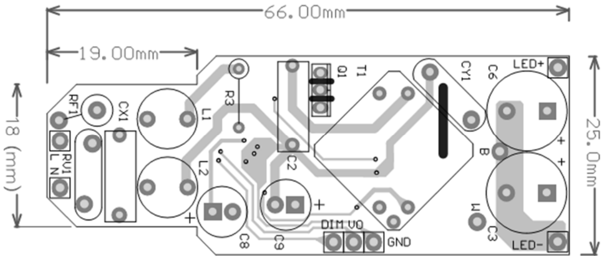
Bottom layer
