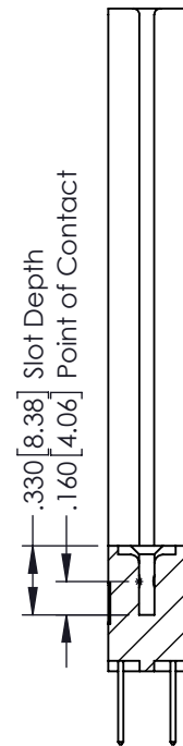
SECTION A-A
