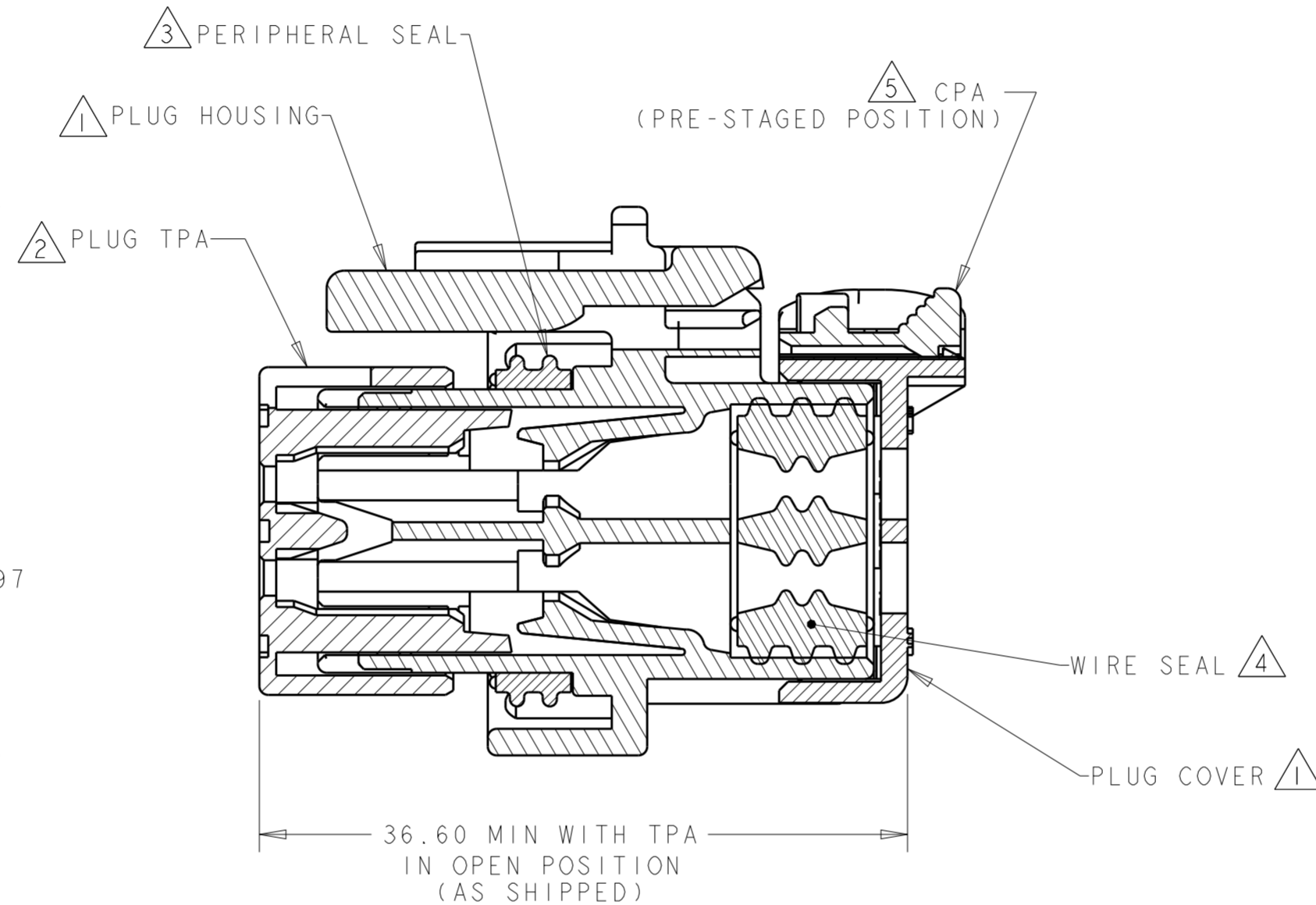
SECTION A-A
