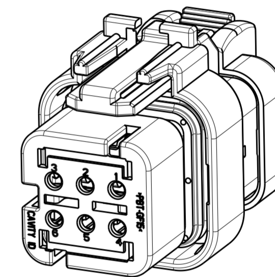
SCALE 2:1
