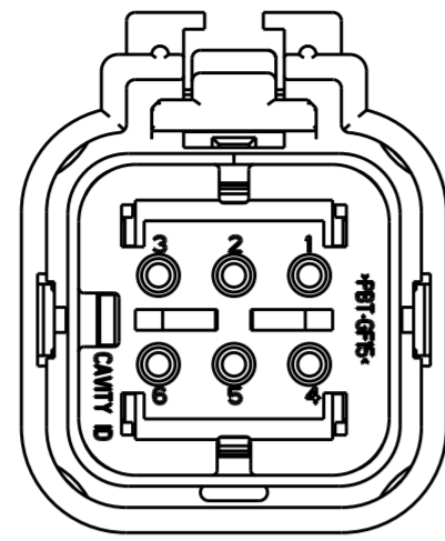
2098237-3 BLUE TPA KEY C SCALE: 2:1
