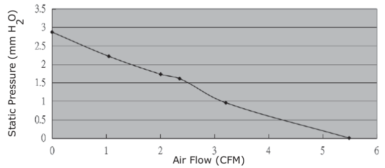
CFM-4010B-065-251
