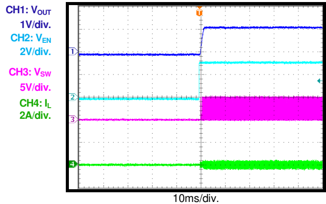
EN On I_{OUT} = 0A, PWM
