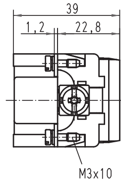
Montageausschnitt panel cut out 1:2
