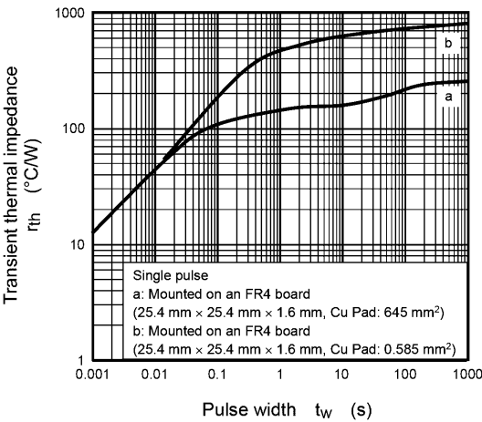
Fig. 8.13 r_{th} - t_w
