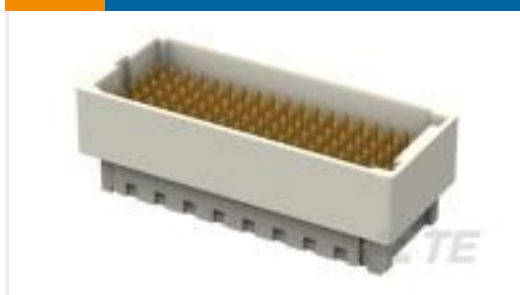
TE Part #2102060-1 Mezalok, Pin, 114 p, 50 Au, TL
