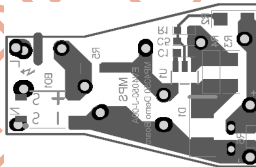
Bottom Layer
