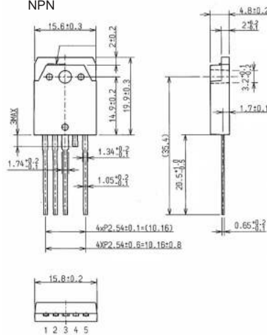
• TO3P-5Pin NPN
