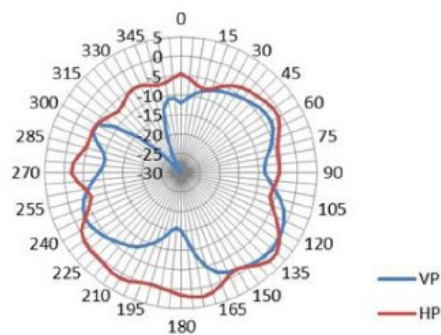
VO Plane
