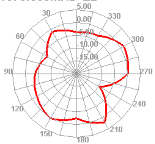
1575.000MHz E2
