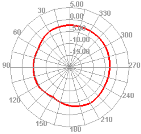
1602.000MHz H
