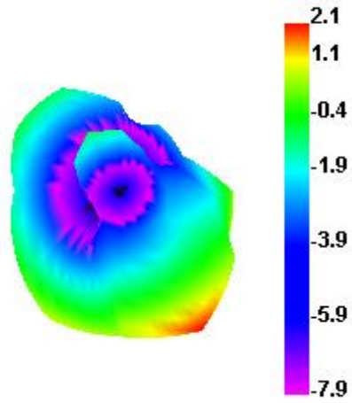
1586.000MHz
