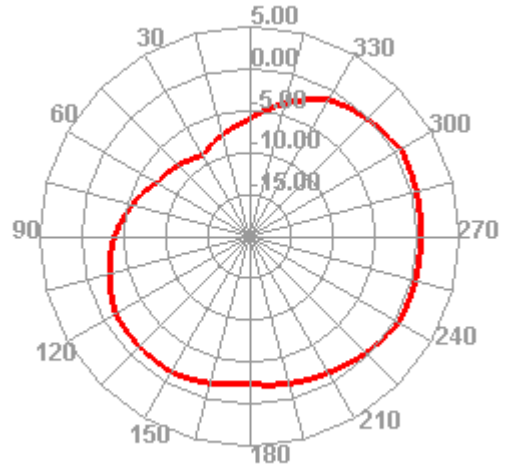
1586.000MHz H
