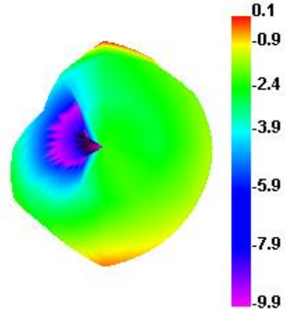
1602.000MHz E2
