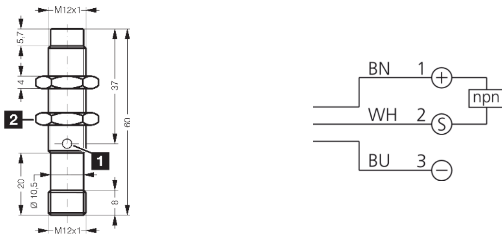
1) LED 2) Schlüsselweite 17 mm BN: braun BU: blau WH: weiß
