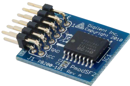
The PmodSF2.
