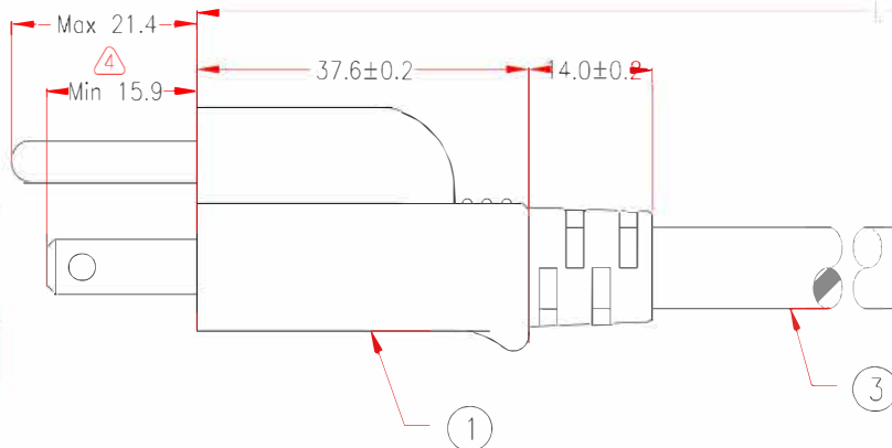
NEMA 5-15P( MSL-105)
