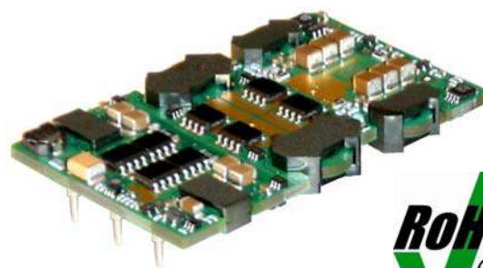
QD48T012025 Converter
