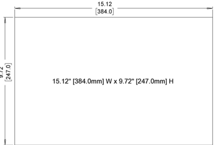
Cutout Dimensions
