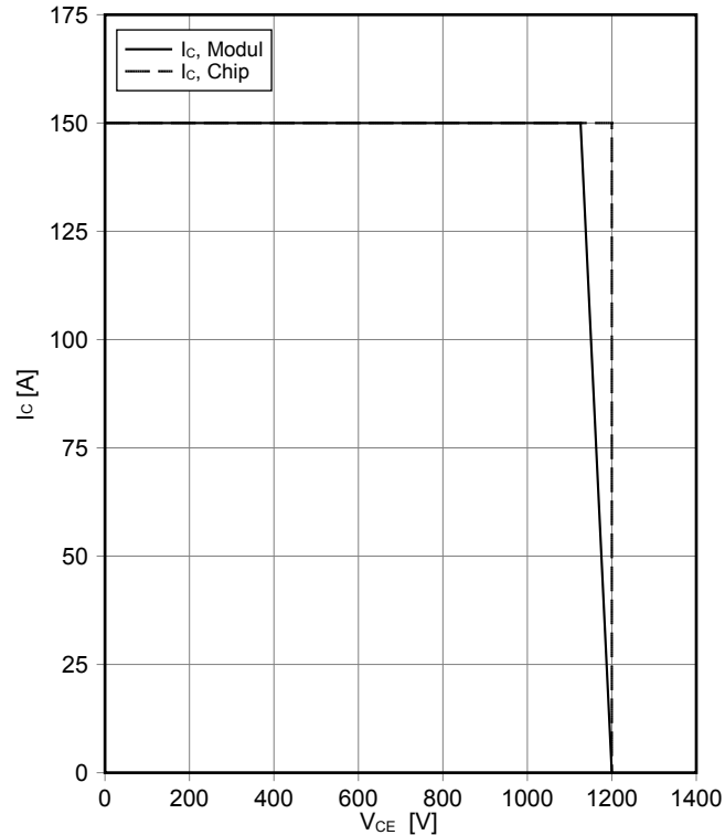
Sicherer Rückwärts-Arbeitsbereich IGBT, Wechselrichter (RBSOA) reverse bias safe operating area IGBT, Inverter (RBSOA) I_C = f(V_{CE}) V_{GE} = \pm 15\text{ V} , R_{Goff} = 2.2\ \Omega , T_{vj} = 175^\circ\text{C}
