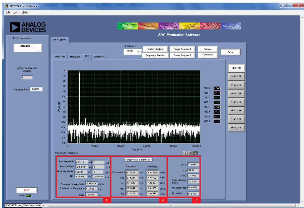
Figure 24. FFT Tab
