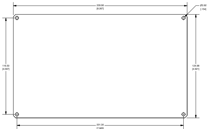
ENCLOSURE LID
