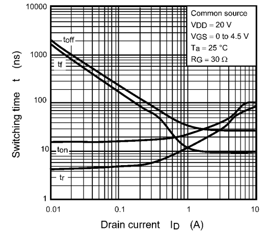
Fig. 8.10 t - I_D
