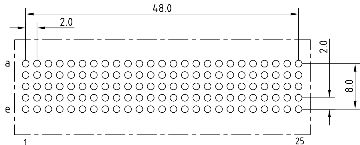
LAY-OUT P.C.B.-HOLE
