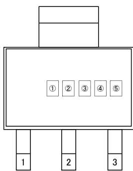
SOT-223
