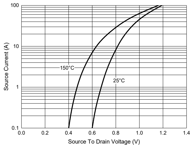
Fig. 6 - I_S - V_{SD}
