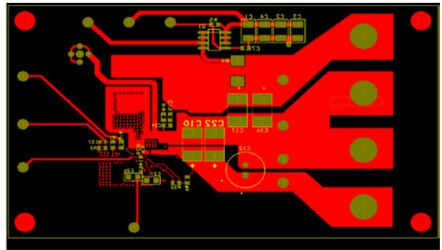
Figure 17. Bottom Layer
