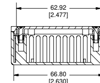
SECTION D-D
