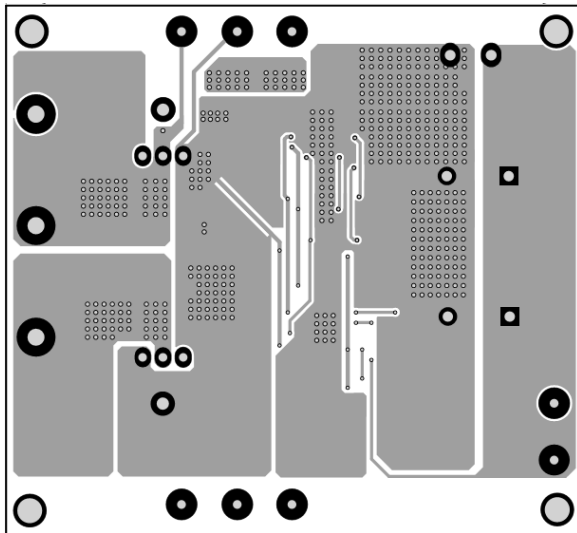
Figure 3—Top Layer
