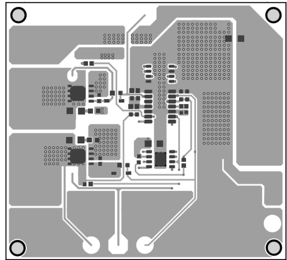
Figure 4—Bottom Layer
