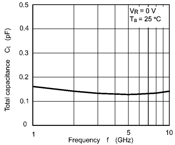
Fig. 9.4 C_t - f
